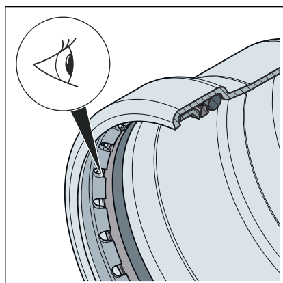
Abb. 11: Schneidring
