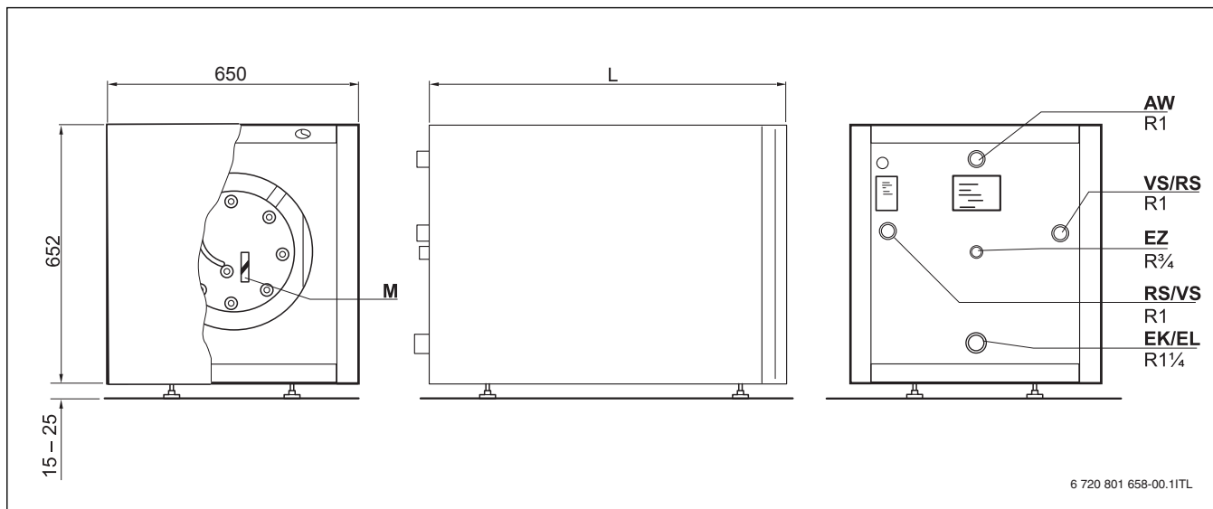
SI.2 Izvedbene i priključne dimenzije WST 135-2 HRC, WST 160-2 HRC i WST 200-2 HRC
