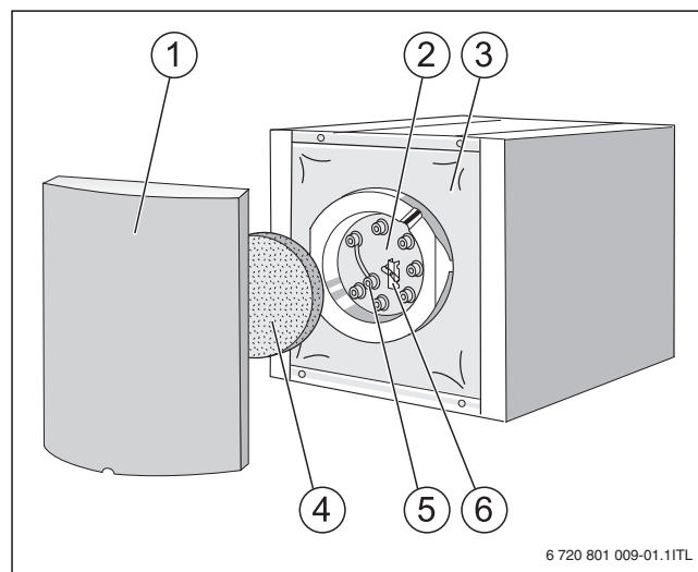
SI.1 WST 135-2 HRC, WST 160-2 HRC i WST 200-2 HRC
