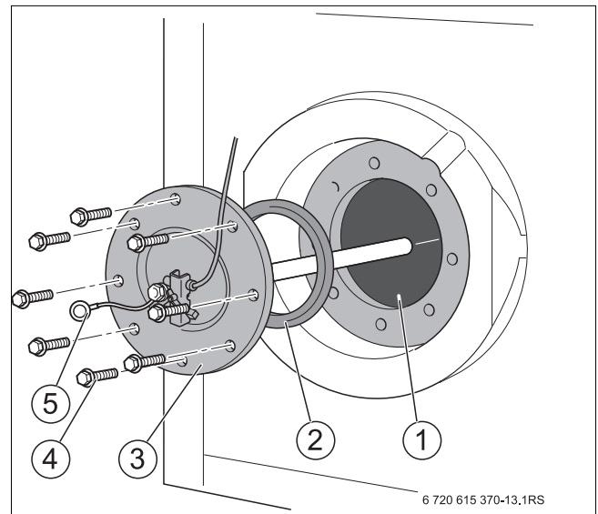
Sl.16 Zatvorite otvor za ispitivanje
