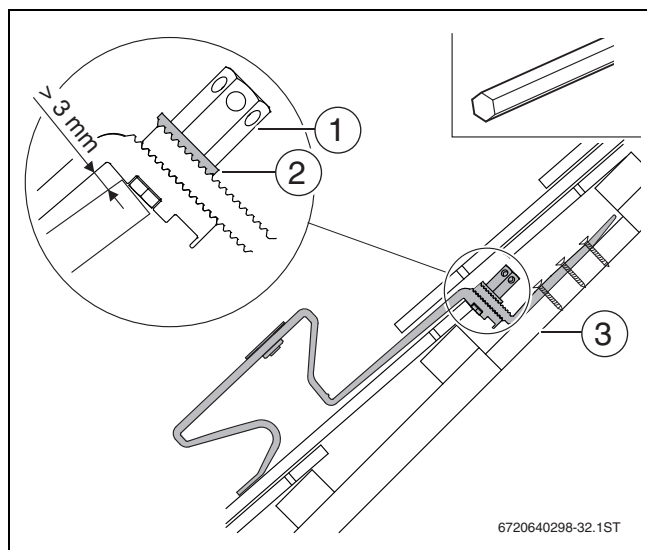
Bild 20 Sparrenanker montieren
