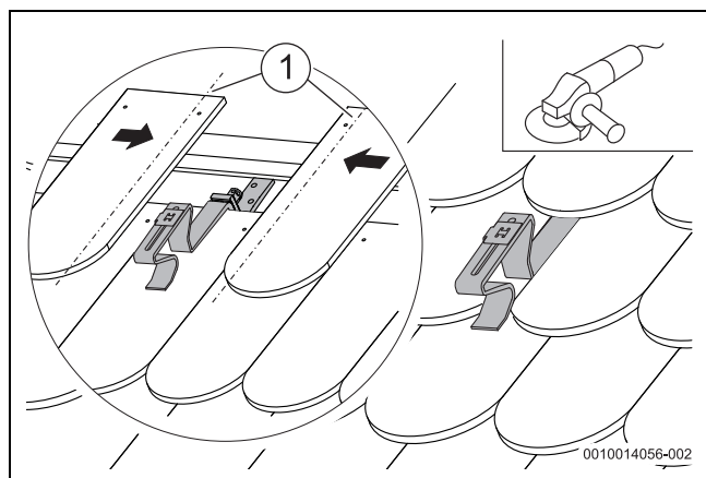
Bild 21 Biberschwanzziegel anpassen
