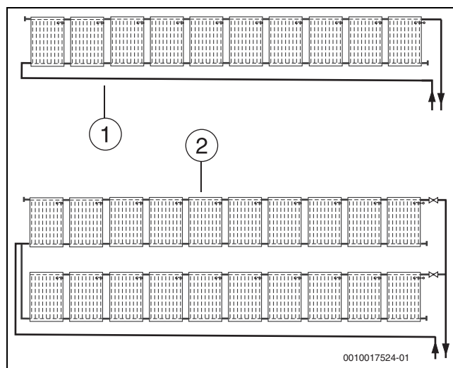
Bild 10 Hydraulischer Anschluss
