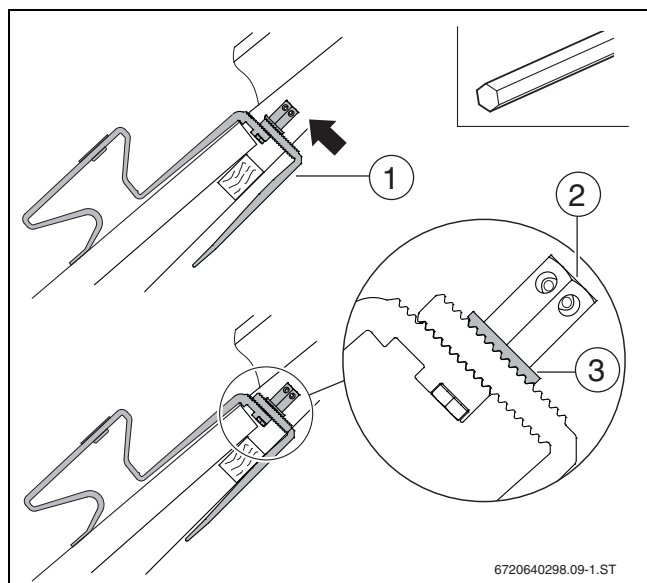
Bild 19 Dachhaken-Unterteil hochschieben
