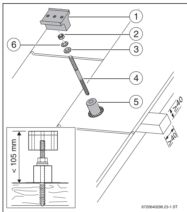
Bild 27 Stockschraube montieren
