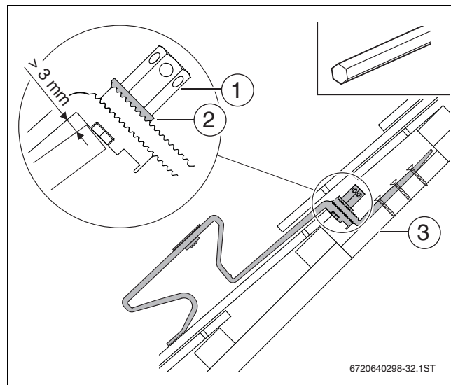
Bild 24 Sparrenanker montieren
