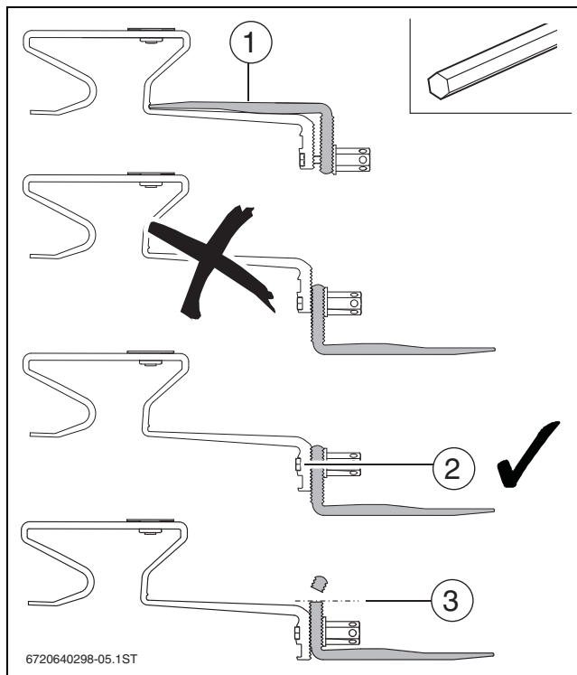
Bild 21 Sparrenanker vorbereiten
