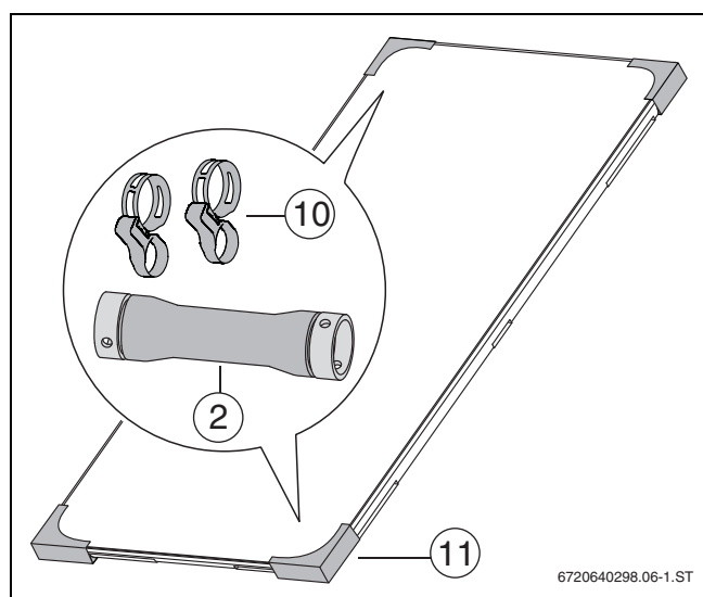
Bild 7 2 Transportschutzzecken beinhalten je 1 Verbindungs-Set (1 Verbindungs-Set enthält 2 Federbandschellen und 1 Solarschlauch)
