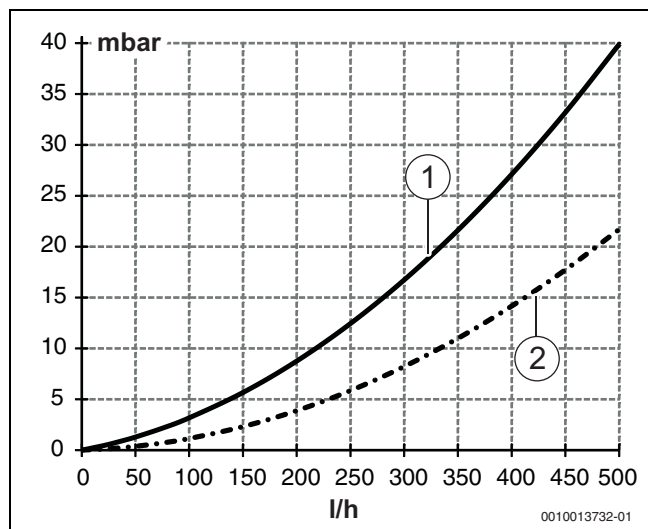
Bild 3 Druckverlustkurve (Wasser-Glykol-Gemisch)
