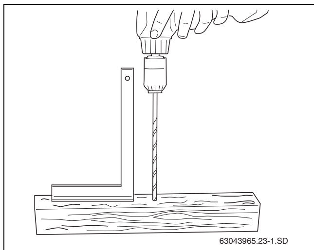
Bild 28 Bohrschablone herstellen
