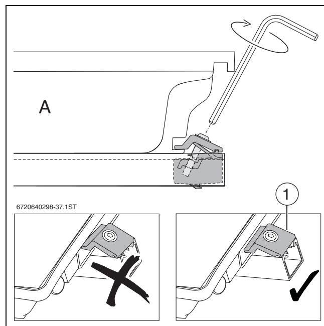
Bild 45 Kollektorspanner festdrehen
