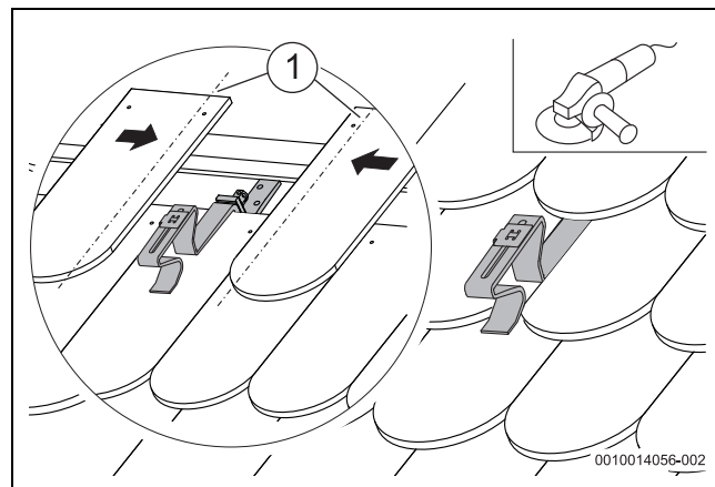
Bild 25 Biberschwanzziegel anpassen
