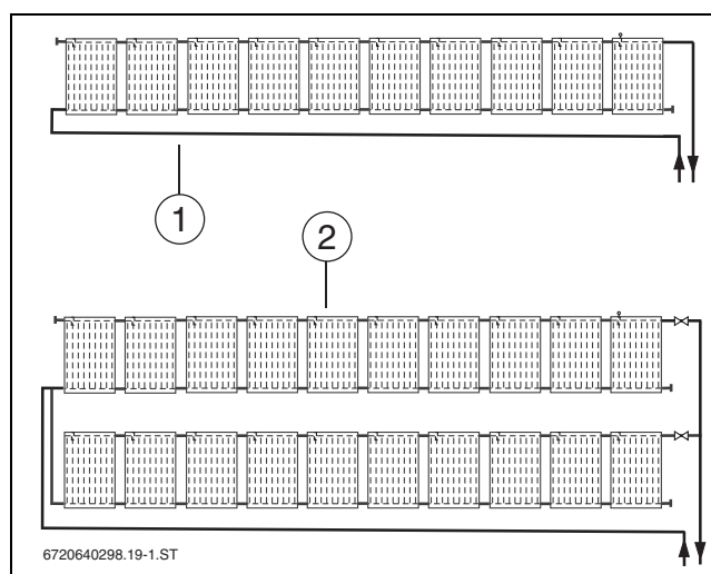
Bild 10 Hydraulischer Anschluss
