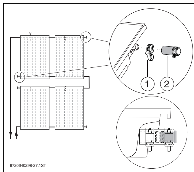
Bild 61 Stopfen montieren
