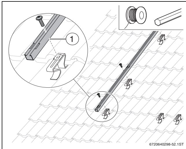
Bild 33 Schneelastprofil montieren
