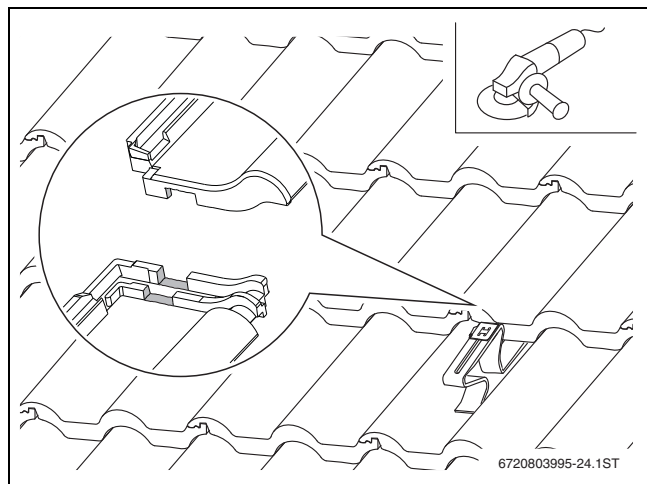
Bild 20 Dachziegel anpassen
