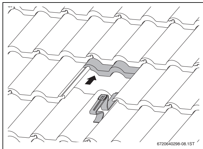
Bild 18 Eingehängter Dachhaken
