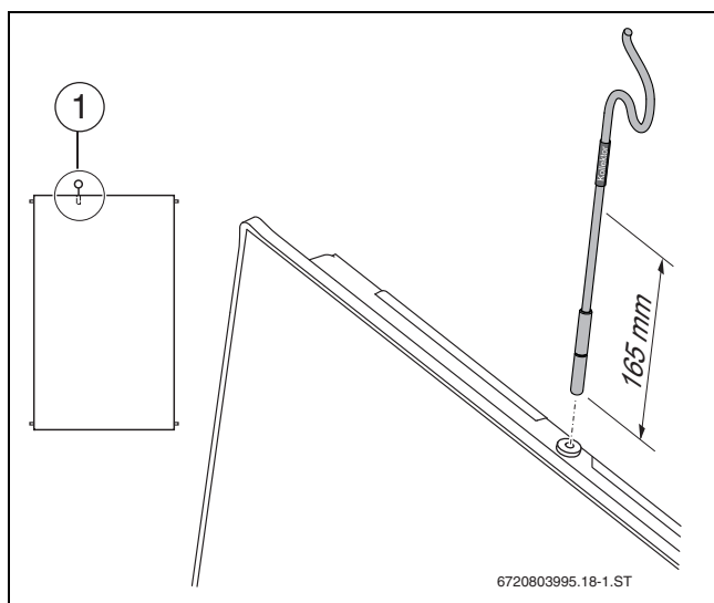
Bild 52 Kollektortemperaturfühler montieren
