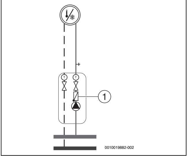
Bild 28 Heizkreis
