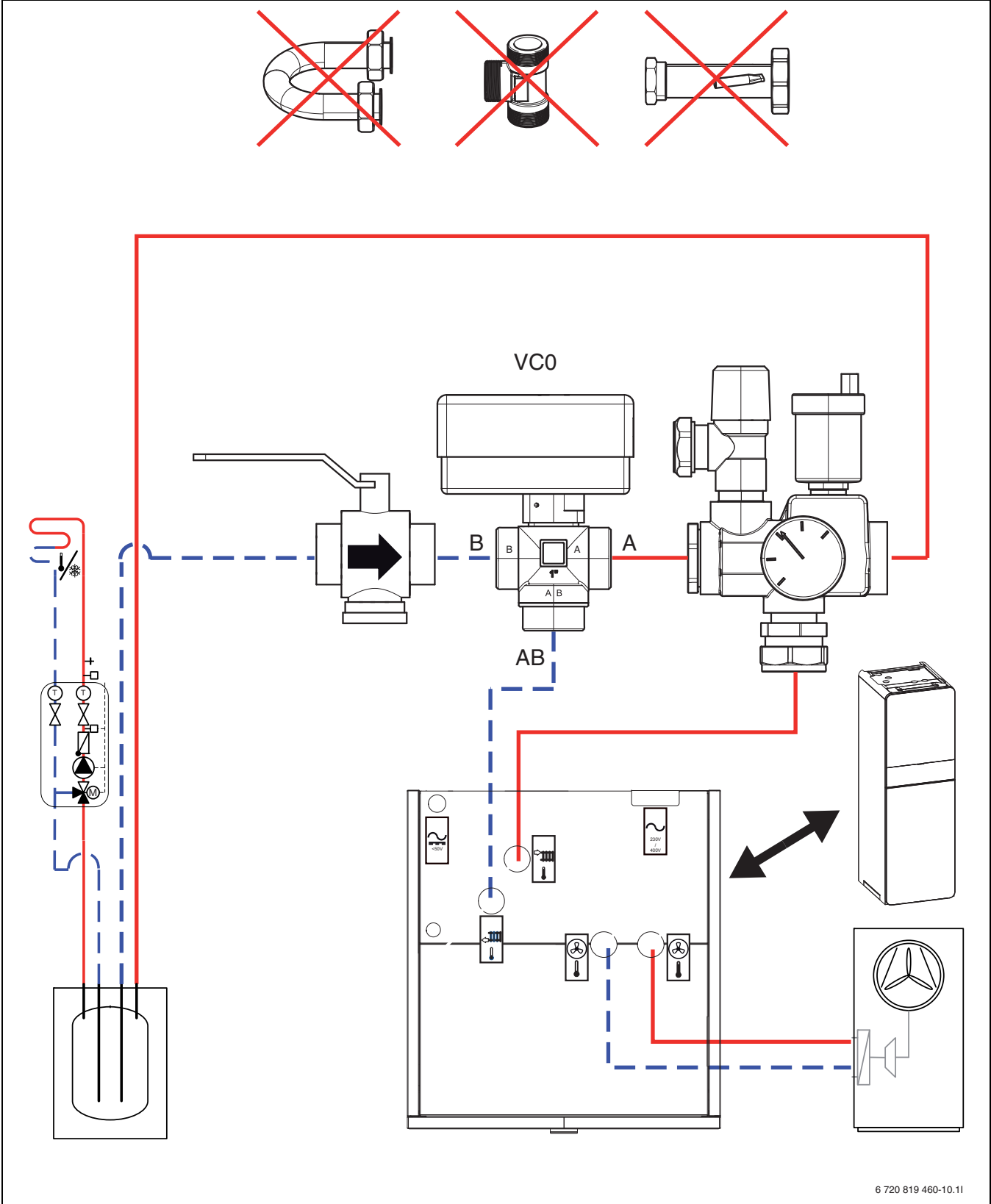
Bild 27 Installation mit Pufferspeicher
