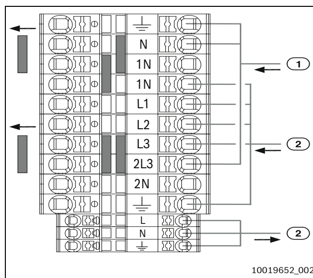
Bild 35 Klemmenanschlüsse und Anordnung der Brücken
