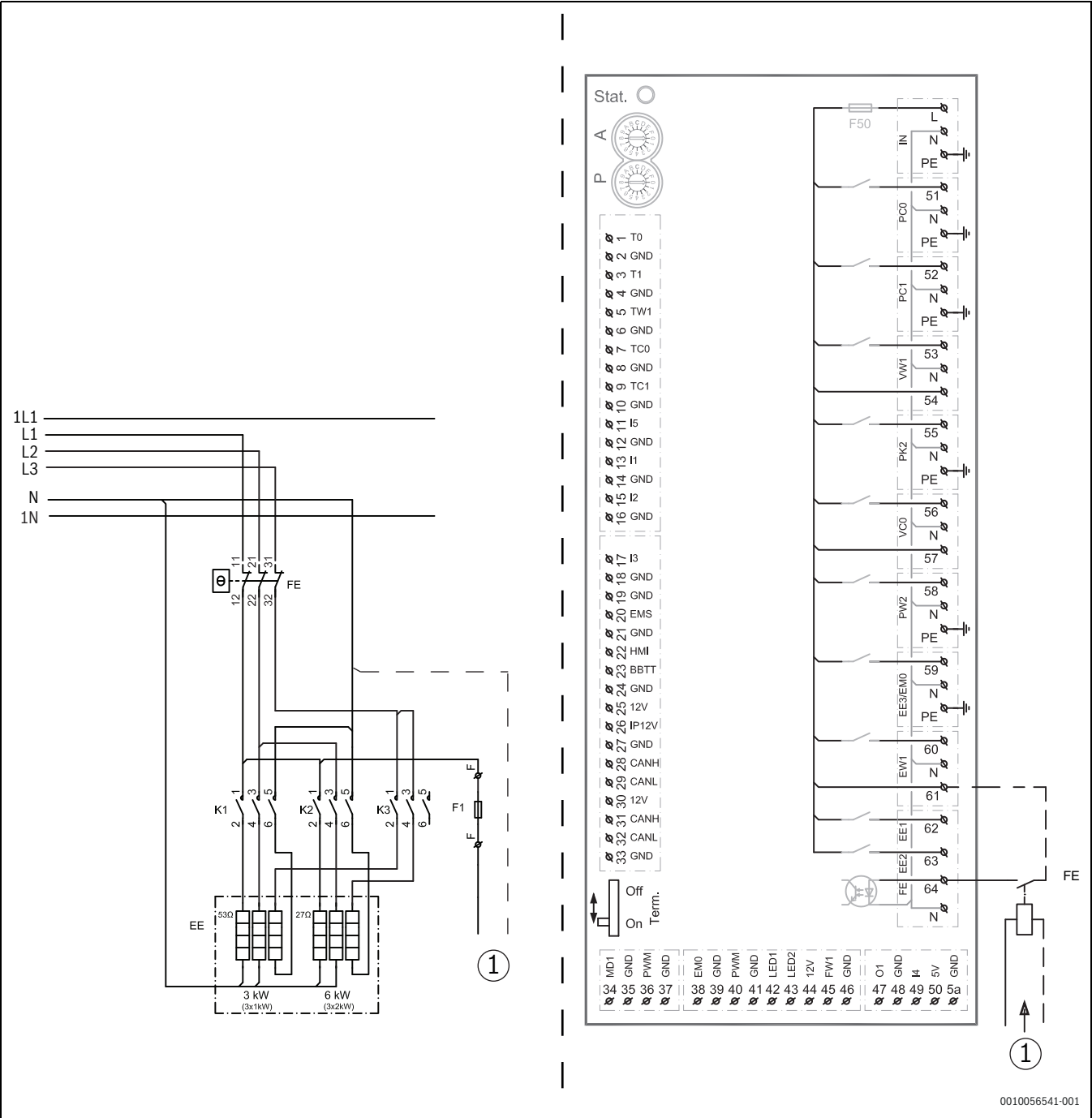
Bild 36 Verdrahtung des zusätzlichen Relais
