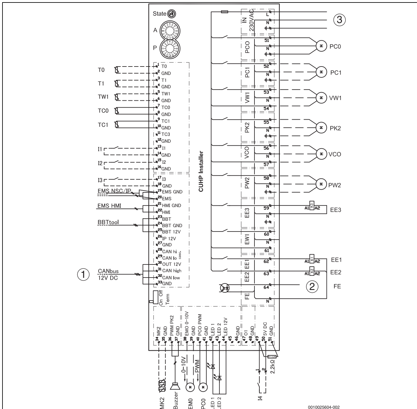
Bild 36 Schaltplan Installationsmodul mit integriertem elektrischen Zuheizer
