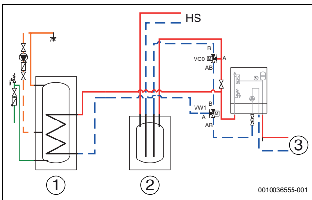
Bild 29 Puffer, VC0-Bypassventil
