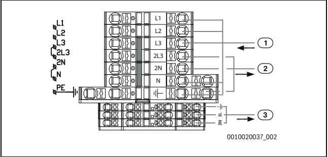
Bild 12 Elektrischer Standardanschluss bei integriertem elektrischen Zuheiz
