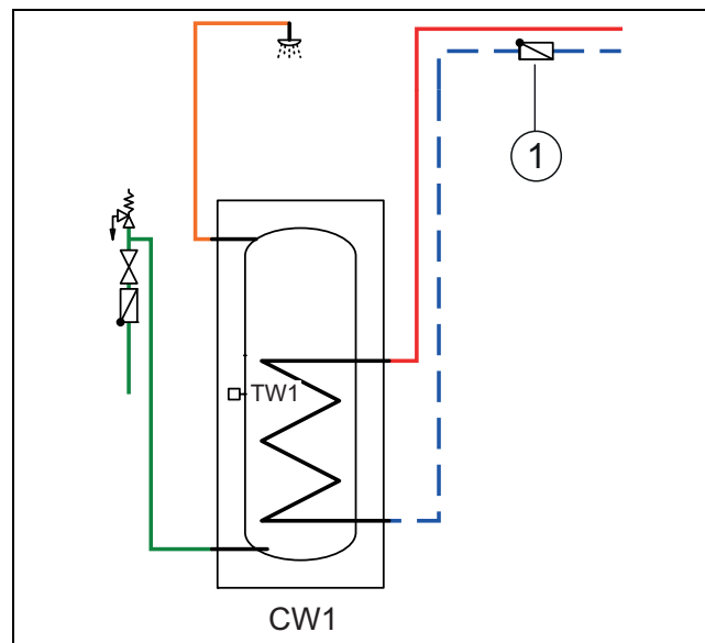
Bild 23 Warmwasserspeicher
