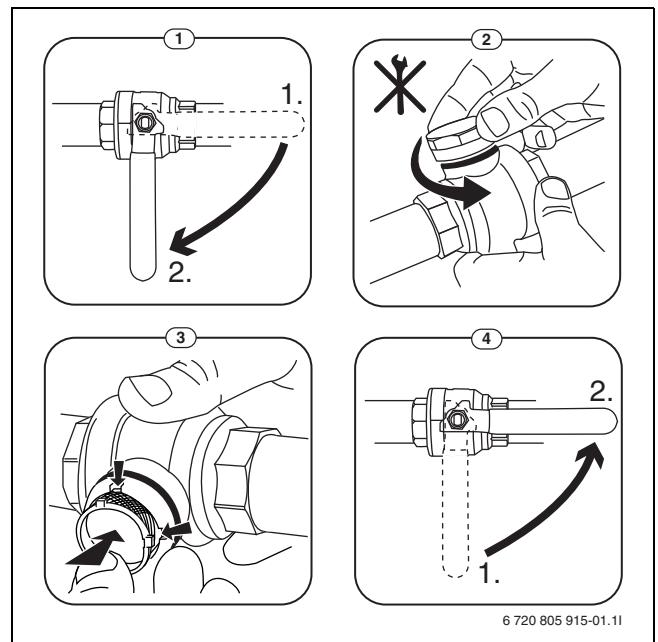
Bild 21 Siebreinigung
