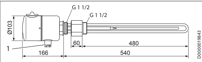
1 Ввод для электропроводки
