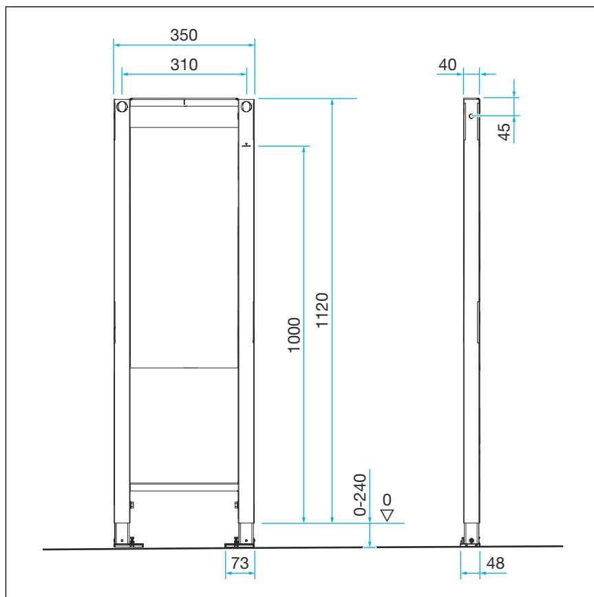
Abb. 2: Abmessungen Modell 8570.31
