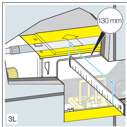
■ UP-Spülkasten 3L
