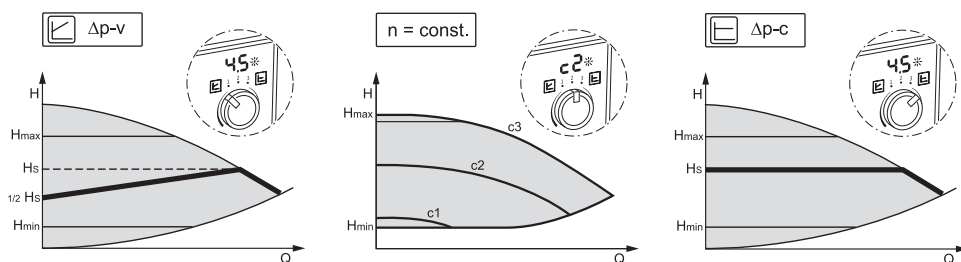
Fig. 4: Sélection du mode de fonctionnement
