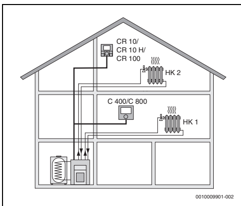
Bild 2 CR 10/CR 10 H/CR 100 als Fernbedienung für den zweiten Heizkreis (HK 2) und C 400/C 800 als Regler für den ersten Heizkreis (HK 1)
