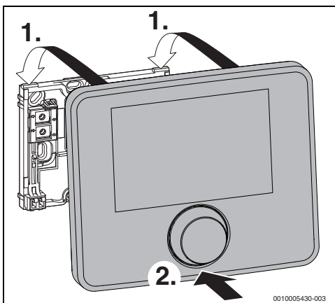
Bild 8 Bedieneinheit einhängen
