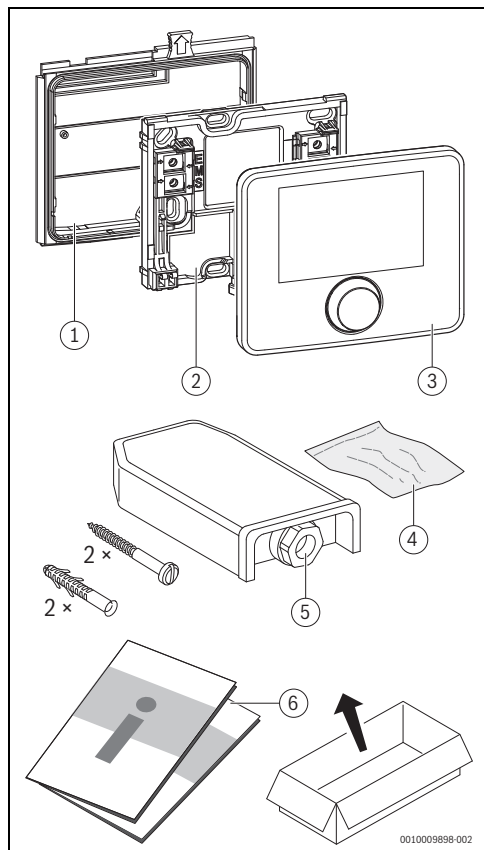
Bild 3 Lieferumfang
