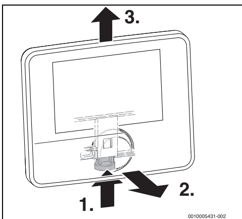
Bild 9 Bedieneinheit abnehmen
