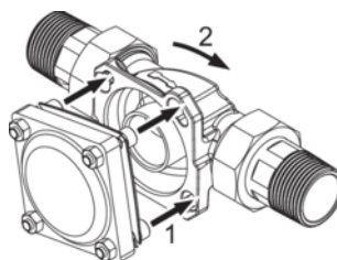
Abb. 8: Schrauben durchführen und einrasten
