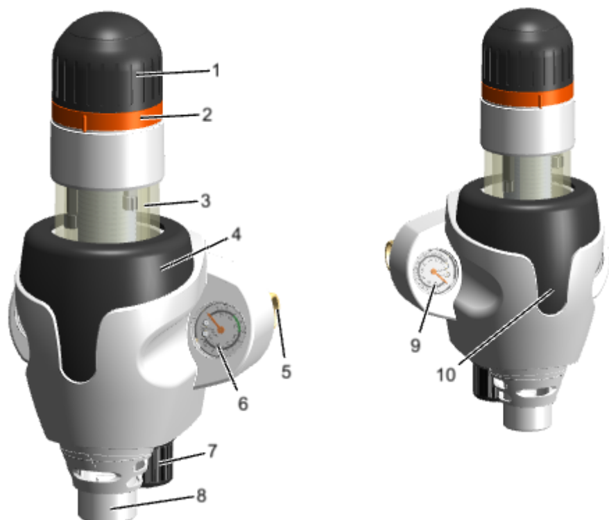
Abb. 1: Funktionsbeschreibung
