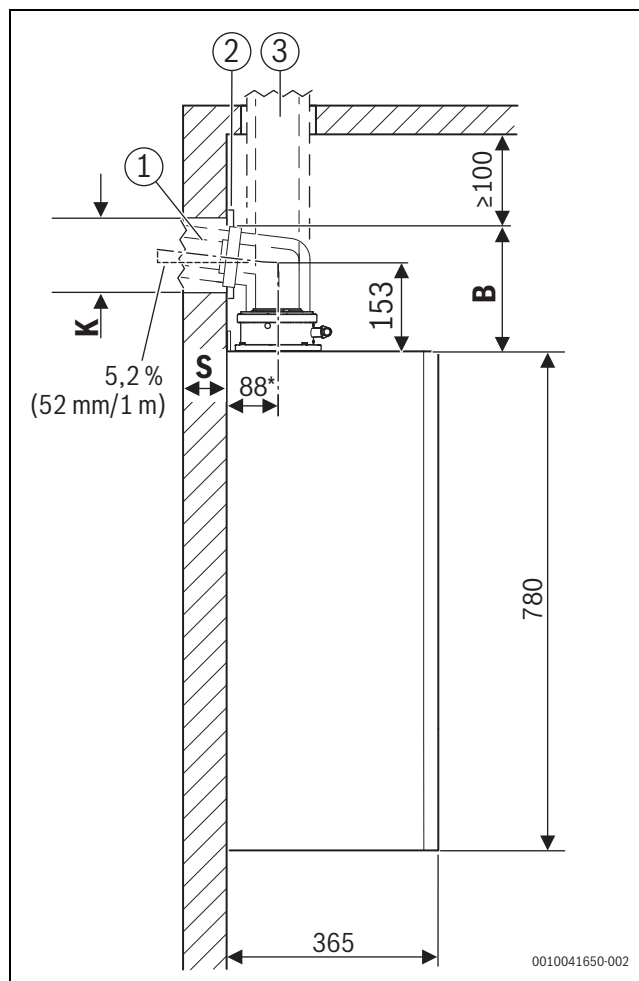
Bild 1 Seitenansicht (mm)
