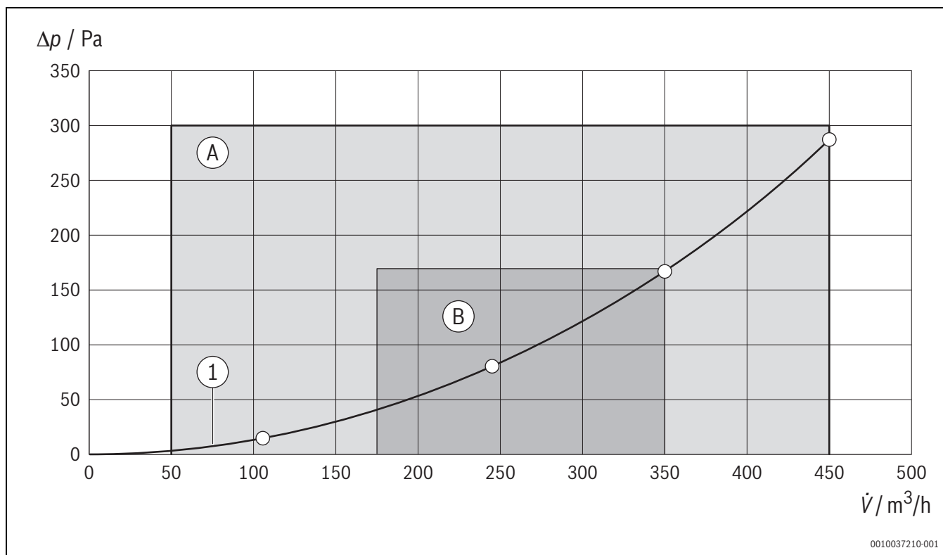
Bild 71 V5001C 450 und V5001C 450 E Kennlinien Druckerhöhung/Volumenstrom (Lüftungsstufen nach DIN 1946-6)
