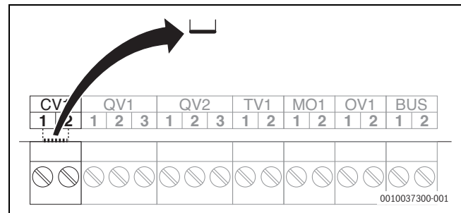
Bild 29 Brücke entfernen
