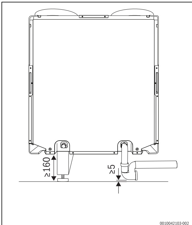
Bild 36 Mindestabstände V5001C... mit Bodenkonsole HRV-FMS und angeschlossenem Kugelsiphon HRV-BS
