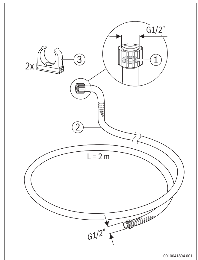
Bild 37 Schlauchsiphon-Anschluss-Set
