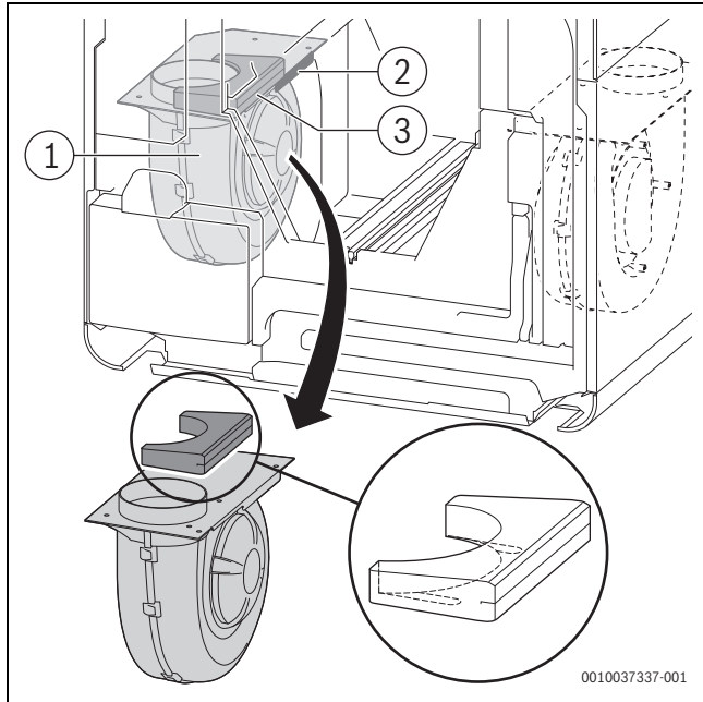
Bild 62 Gebläse herausziehen
