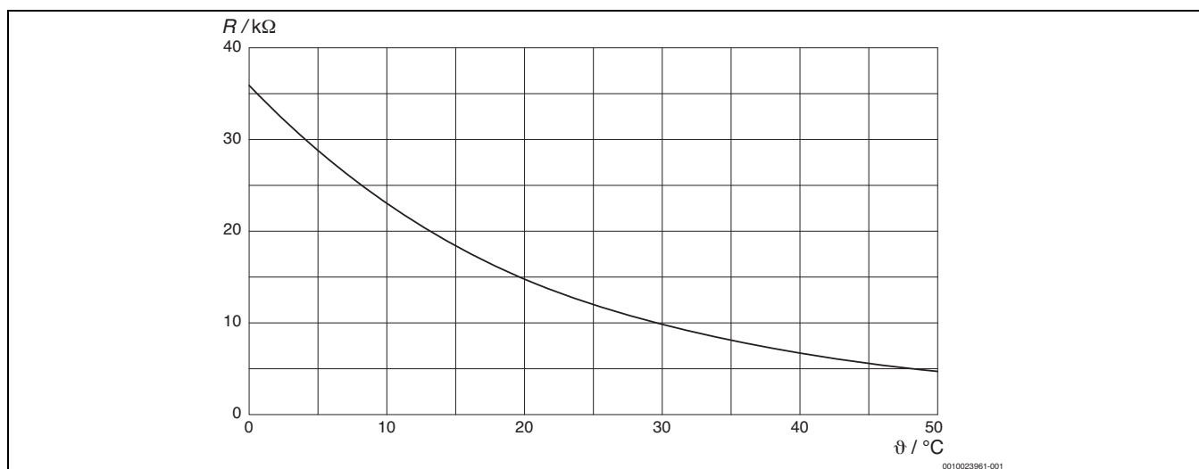
Bild 69 Kennlinie TV1 (12K)
