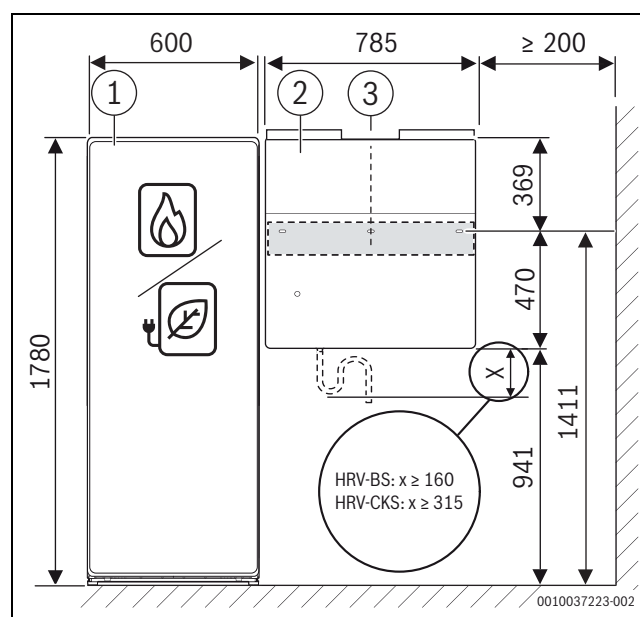
Bild 33 Einbaumaße im System mit einem Bosch Wärmeerzeuger
