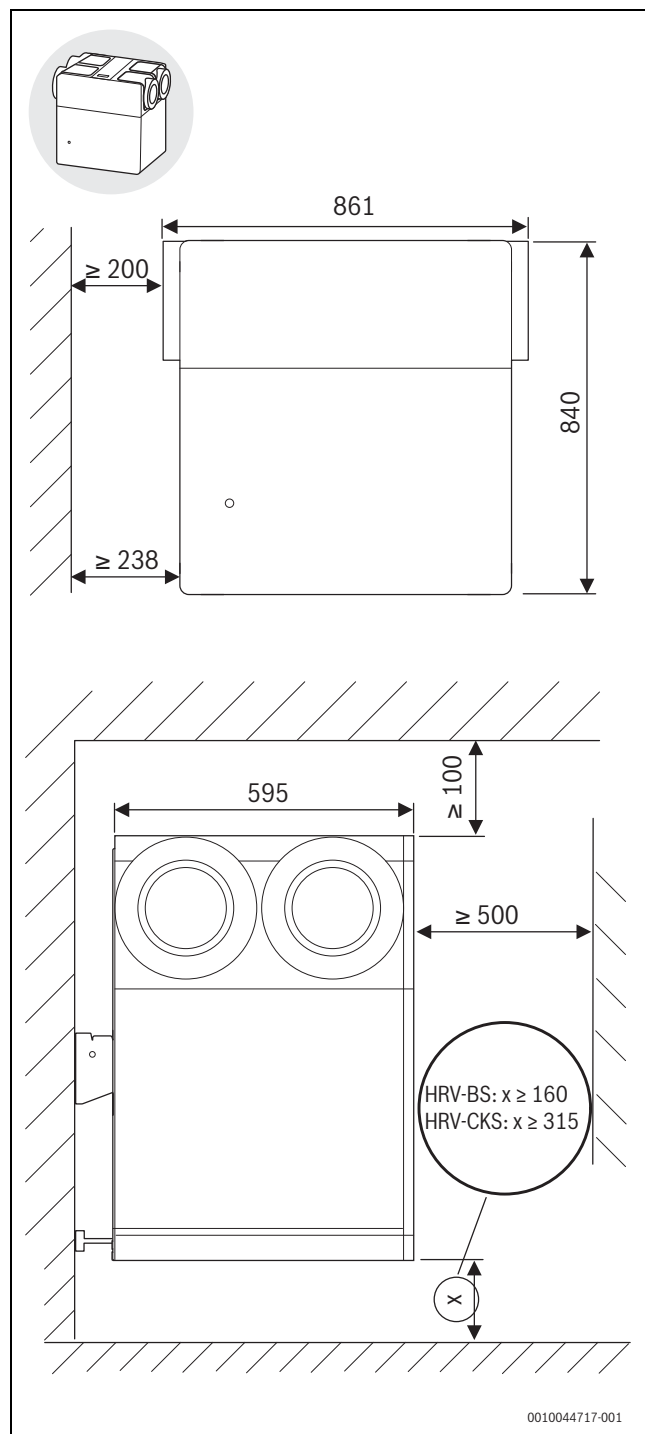
Bild 4 Abmessungen und Mindestabstände Wandinstallation V5001C... - Mindestabstände wenn Anschlussstutzen waagrecht
