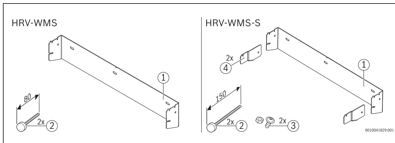
Bild 31 Lieferumfang HRV-WMS/HRV-WMS-S
