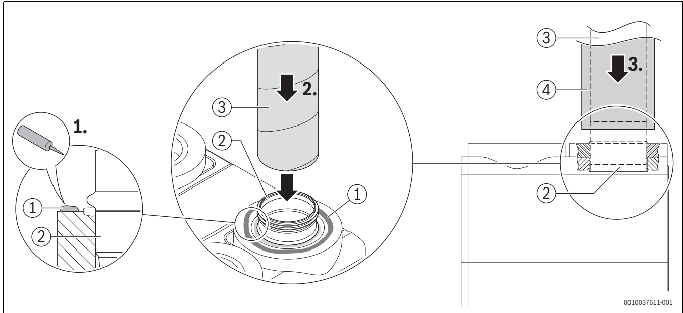
Bild 44 Aufbau Luftrohranschluss
