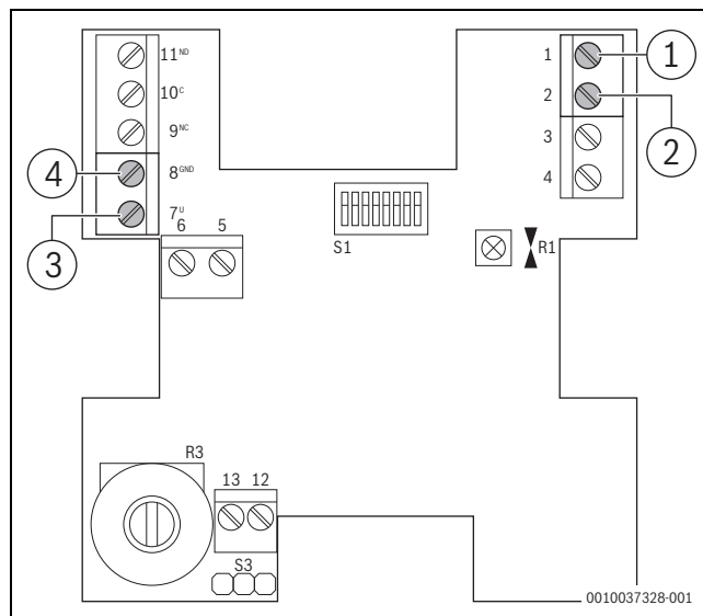
Bild 54 Interne elektrische Anschlüsse CS/VS-R
