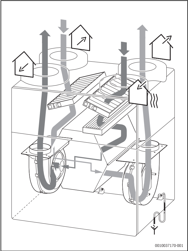
Bild 9 Luftseitiger Geräteanschluss (Variante A)
