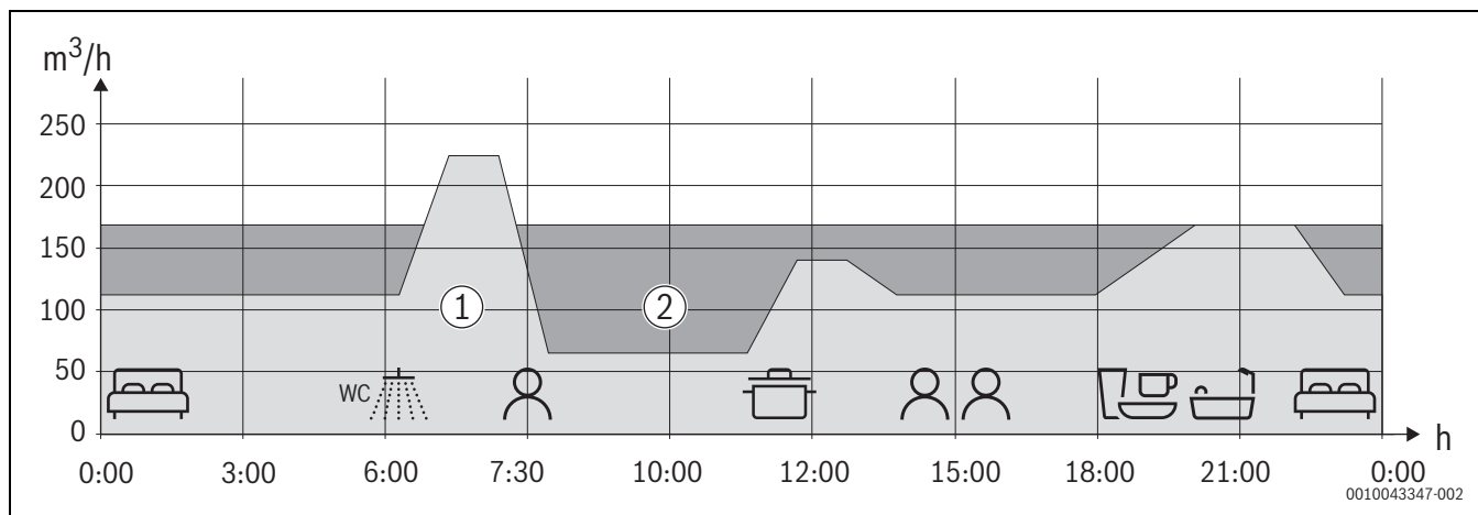
Bild 12 Beispielhafter Vergleich der bedarfsgeregelten/manuellen Lüftung
