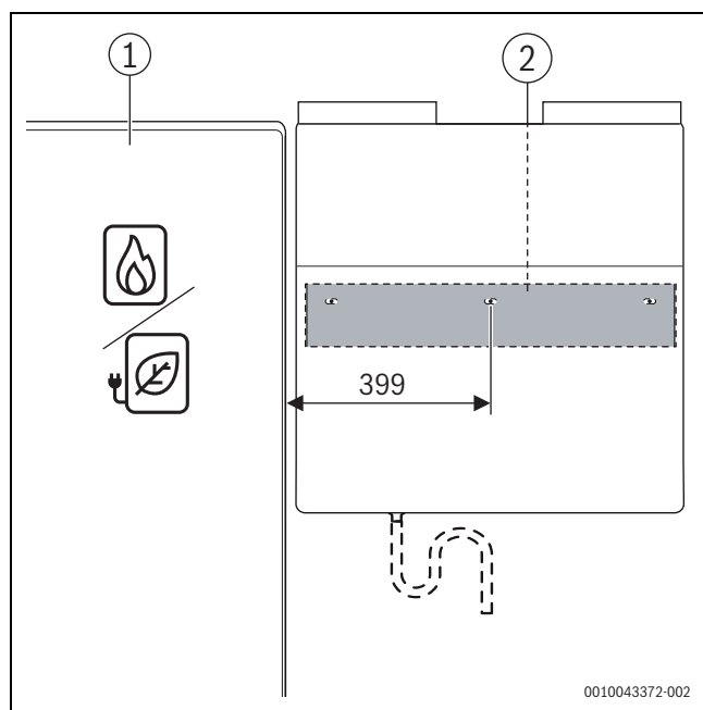
Bild 34 Abstand Bosch Wärmeerzeuger zu V5001C...
