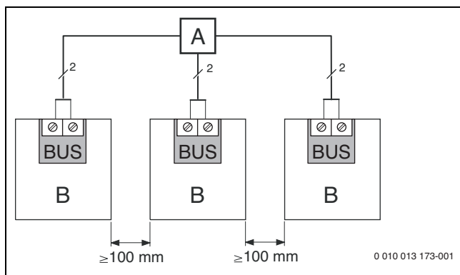
Bild 55 BUS-Verbindungen Leiterquerschnitte
