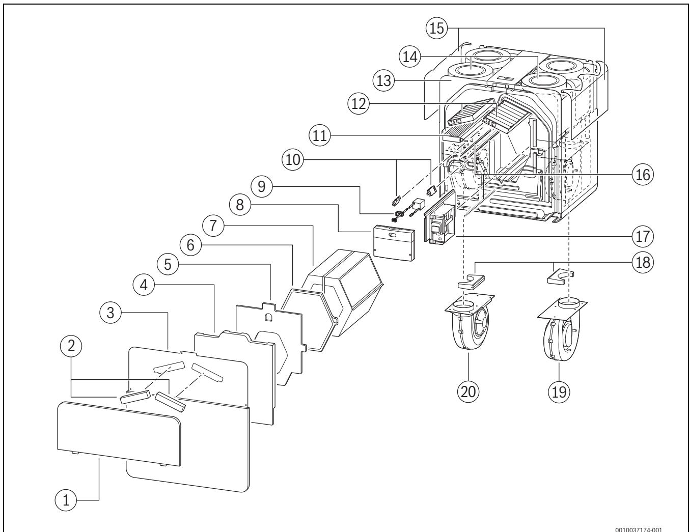
Bild 6 Produktübersicht V5001C...
