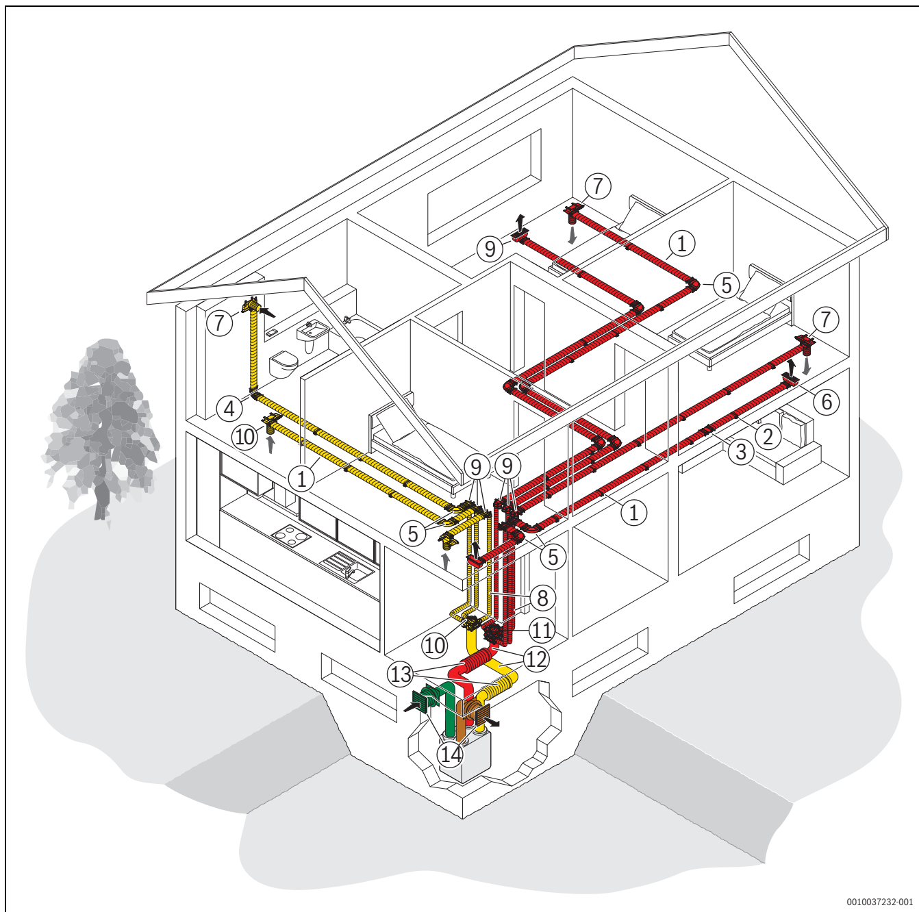
Bild 13 Anlagenbeispiel mit Zubehör
