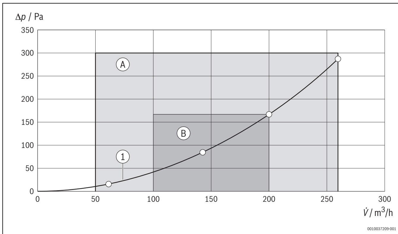
Bild 70 V5001C 260 und V5001C 260 E Kennlinien Druckerhöhung/Volumenstrom (Lüftungsstufen nach DIN 1946-6)
