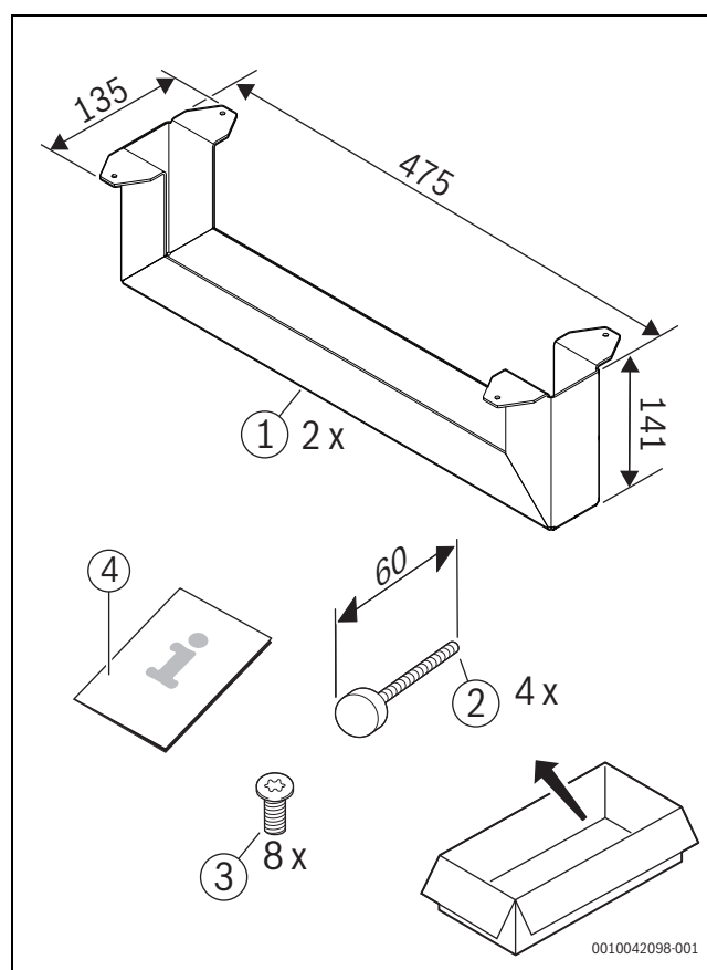
Bild 35 Lieferumfang HRV-FMS
