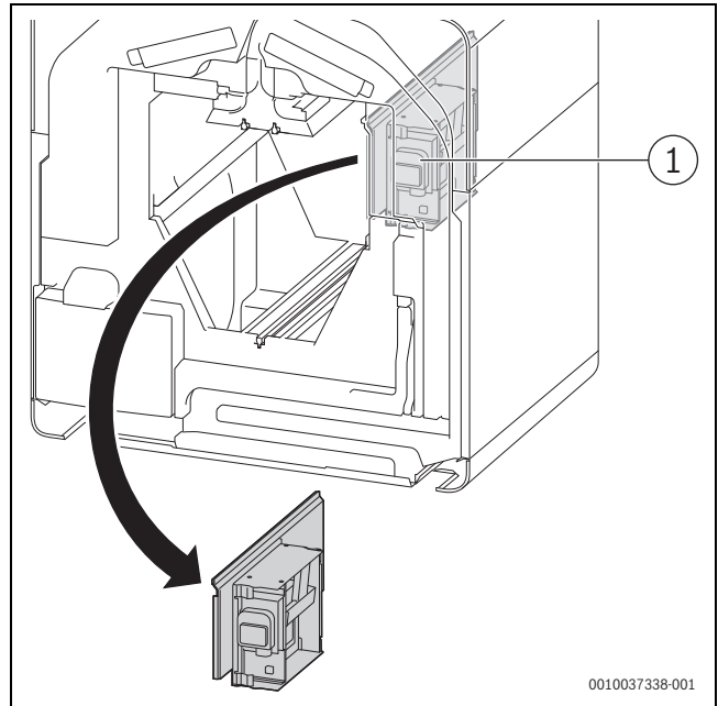
Bild 63 Bypass herausnehmen
