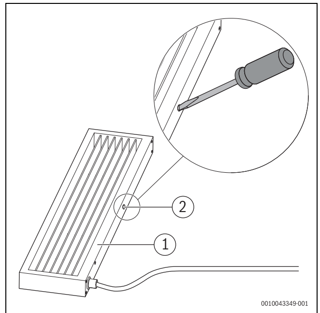
Bild 64 Reset Sicherheitstemperaturbegrenzer des el. Vorheizregisters
