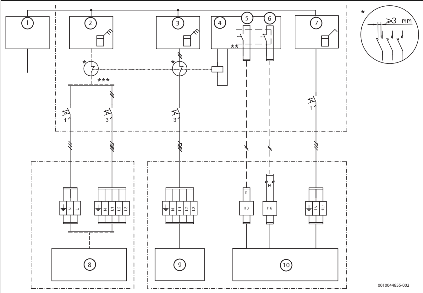
Bild 41 Alternative Lösung
