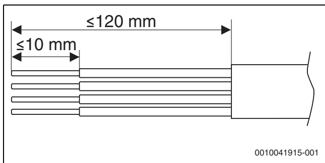
Bild 26 Abisolierung CAN-BUS
