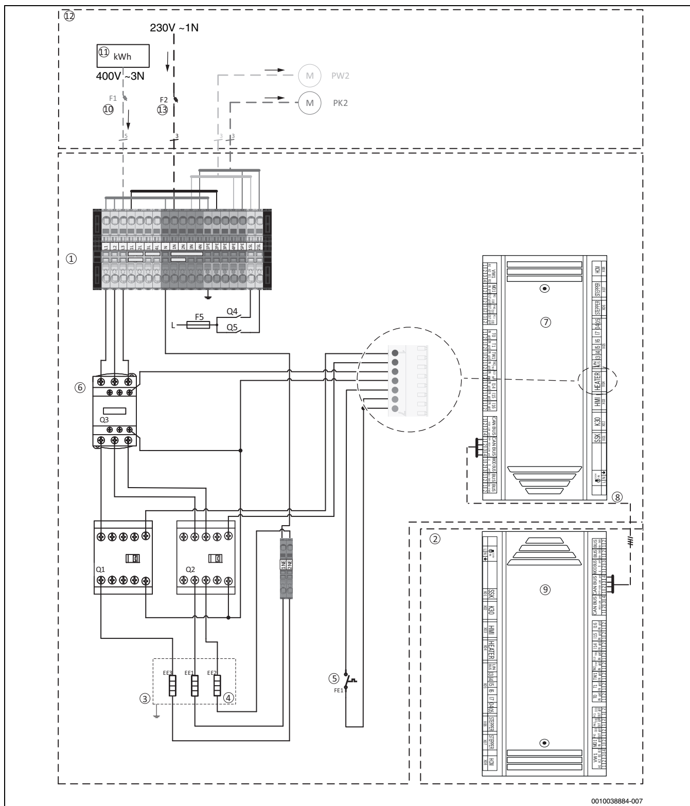
Bild 49 Spannungsversorgung Inneneinheit
