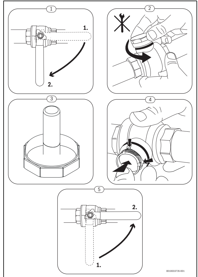
Bild 40 Siebreinigung
