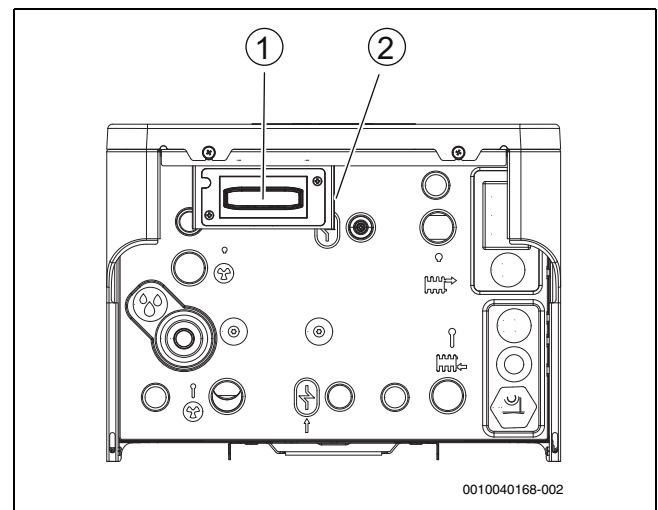
Bild 9 Connect-Key Platzierung
