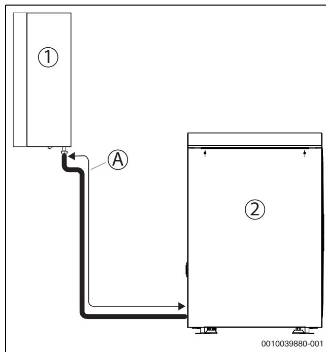
Bild 15 Rohrlänge A
