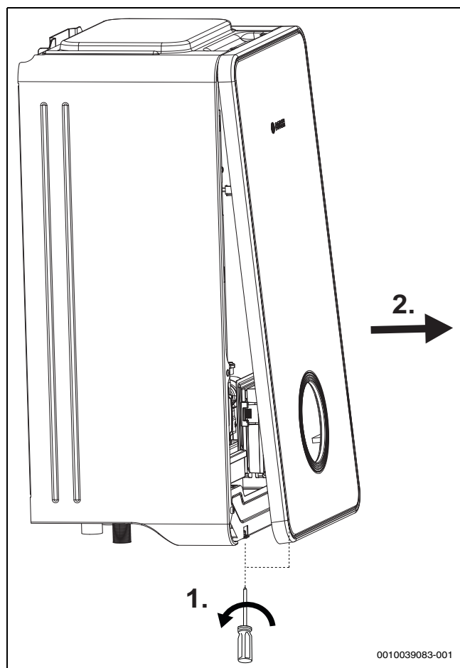
Bild 10 Frontplatten abnehmen
