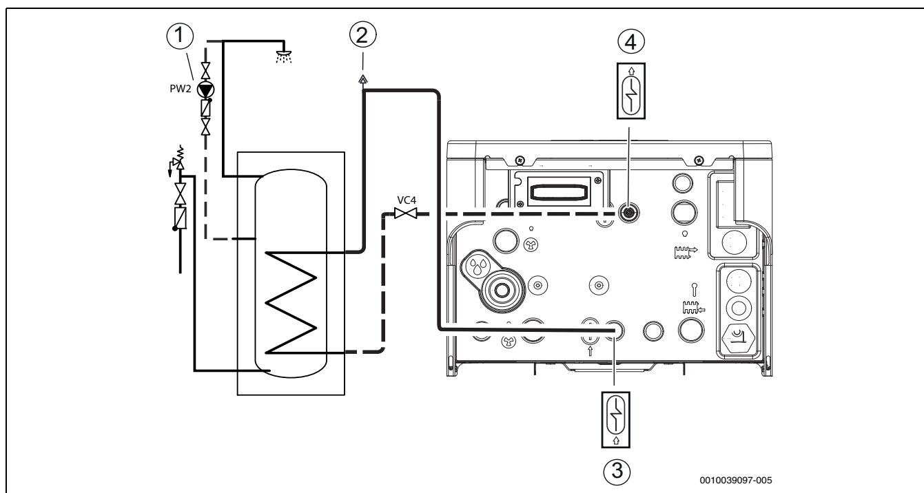
Bild 18 Trinkwasseranschlüsse Inneneinheit
