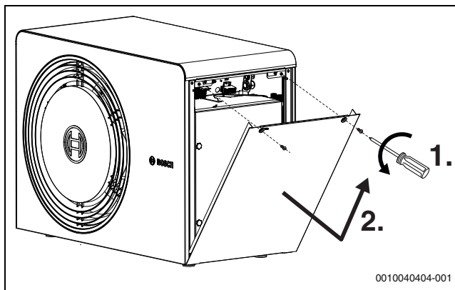
Bild 31 Seitliche Abdeckung
