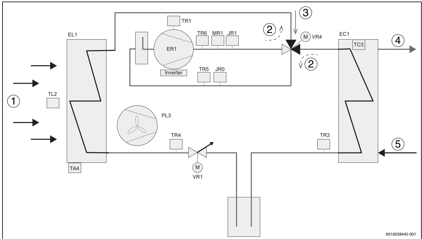
Bild 46 Kältemittelkreis
