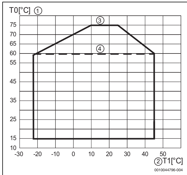
Bild 44 Wärmepumpe im Heizbetrieb ohne Zuheizer
