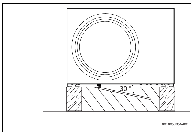
Bild 25 Installation des Kabels für die Tropfschalenheizung
