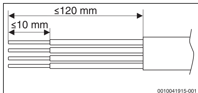
Bild 35 Abisolierung CAN-BUS
