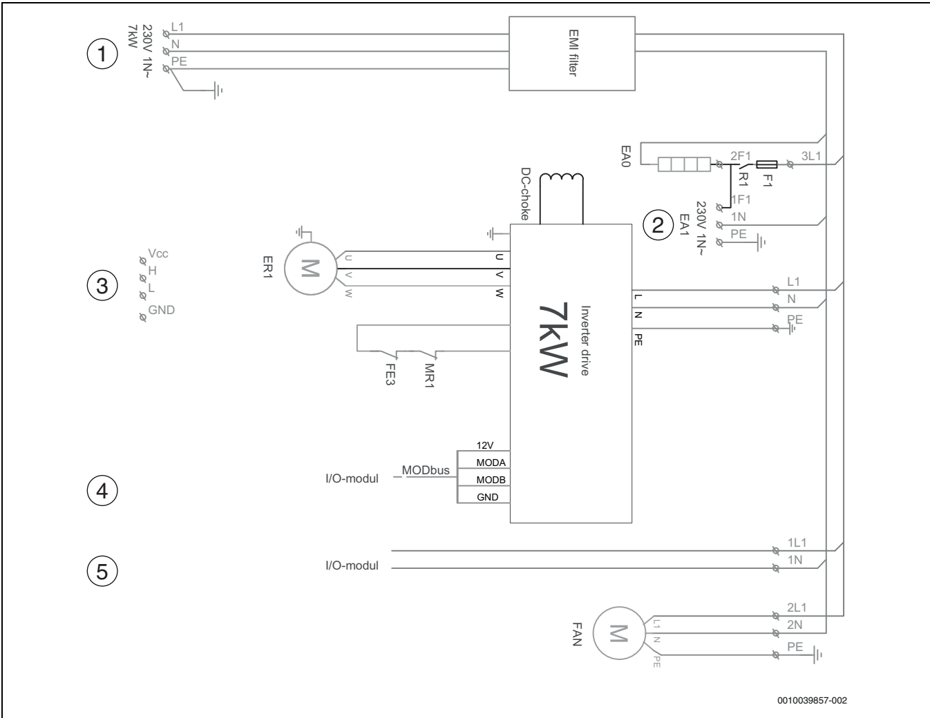
Bild 47 Schaltplan Frequenzumrichter
