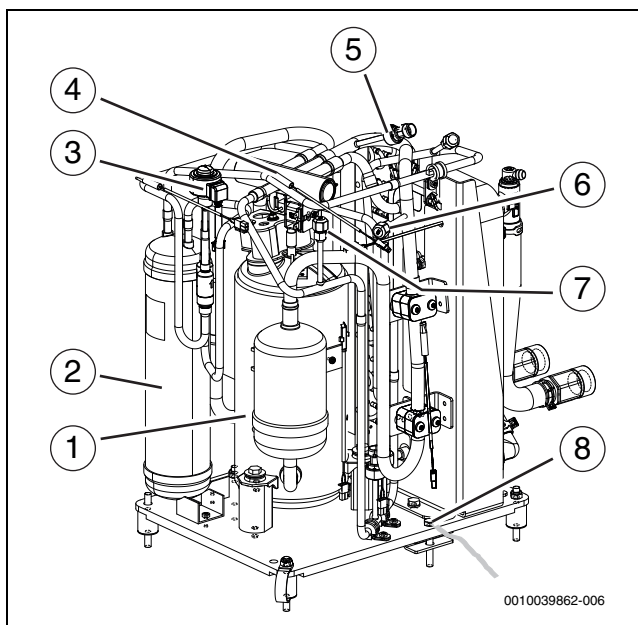
Bild 2 Produktübersicht – Vorderansicht
