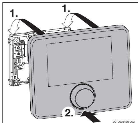
Bild 8 Bedieneinheit einhängen
