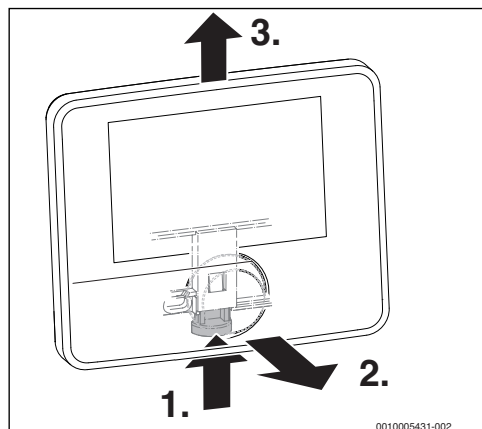
Bild 9 Bedieneinheit abnehmen
