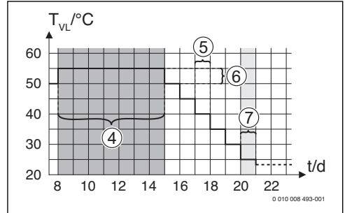
Bild 21 Ablauf der Estrichtrocknung mit den Grundeinstellungen in der Abkühlphase
