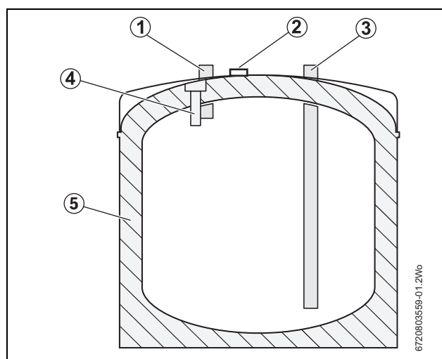
Afb. 1 Primair buffervat
