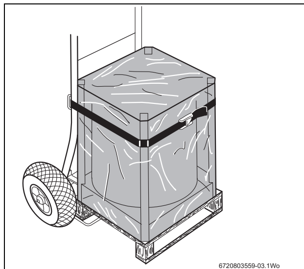
Fig. 3 Transportar el acumulador de agua caliente con el transportador de acumuladores
