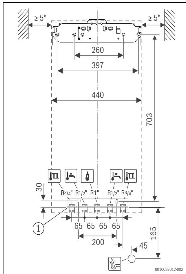
Bild 16 Frontansicht (Maße in mm)
