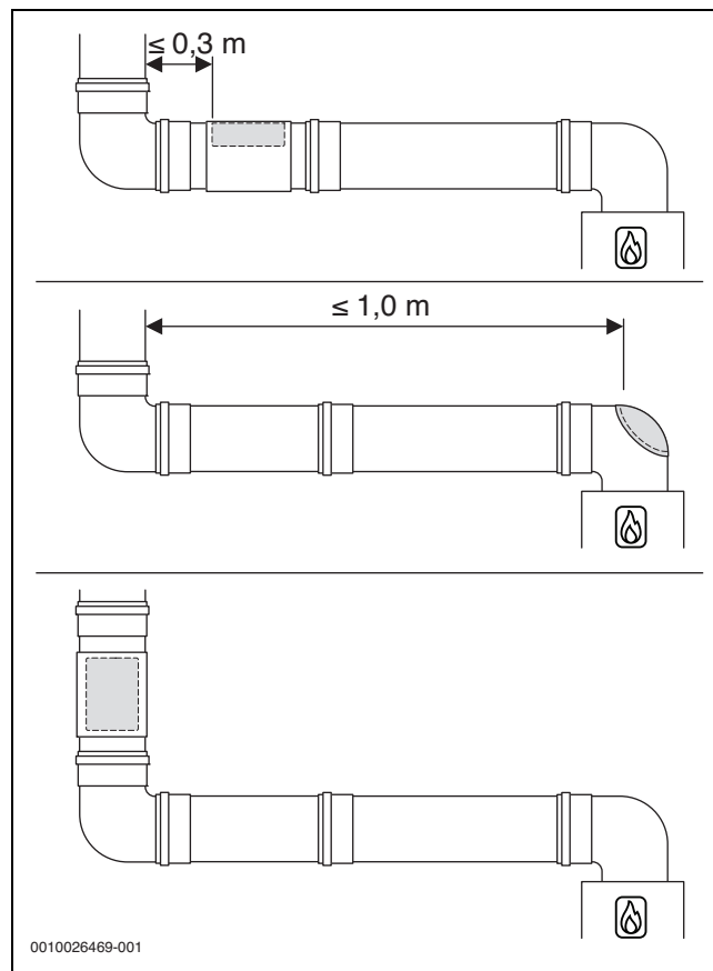
Bild 38 Anordnung der unteren Prüföffnung
