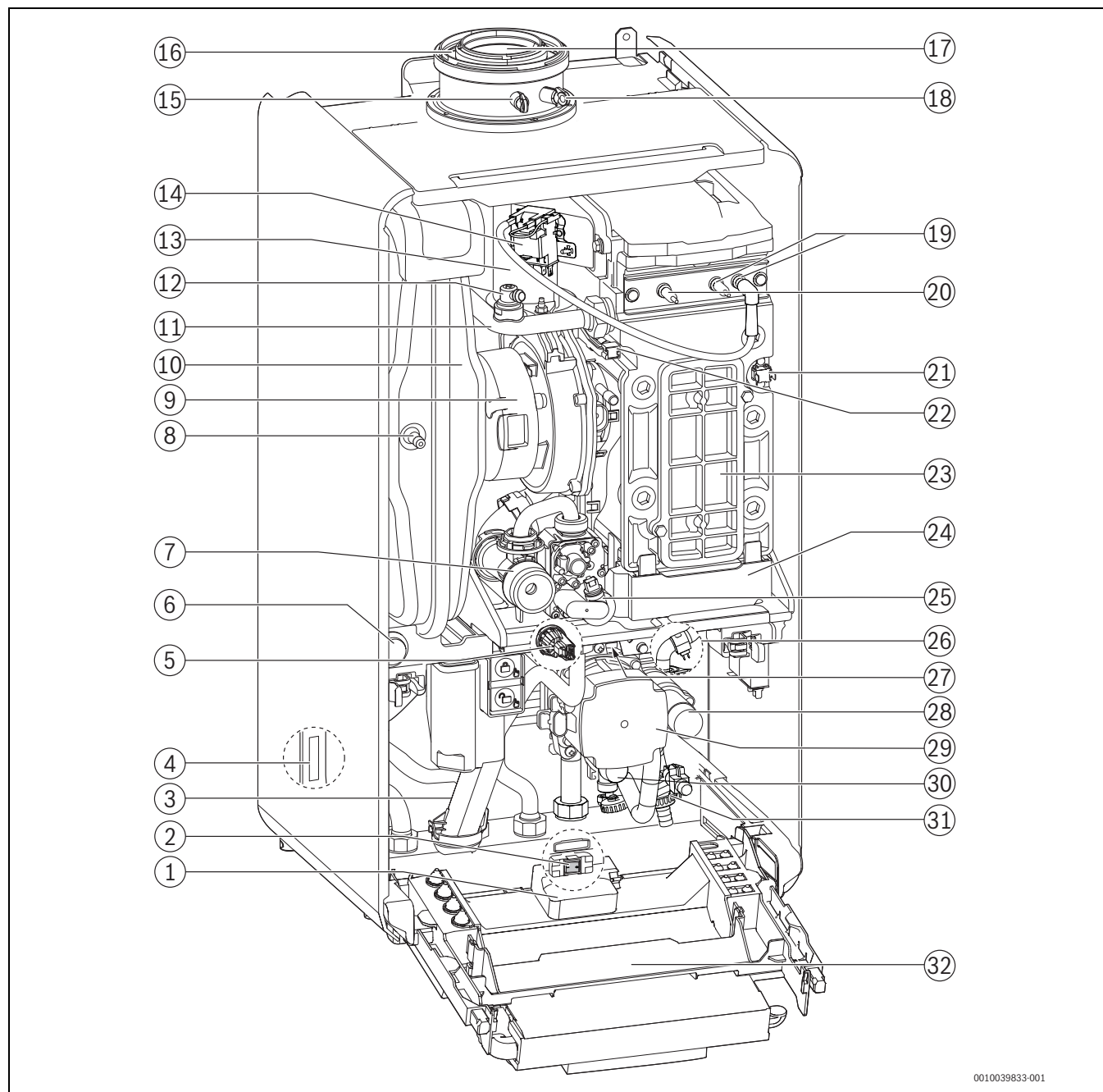
Bild 13 Produktübersicht
