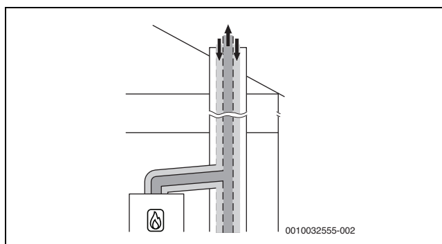
Bild 46 Konzentrische Luft-Abgas-Führung nach C 43x im Aufstellraum
