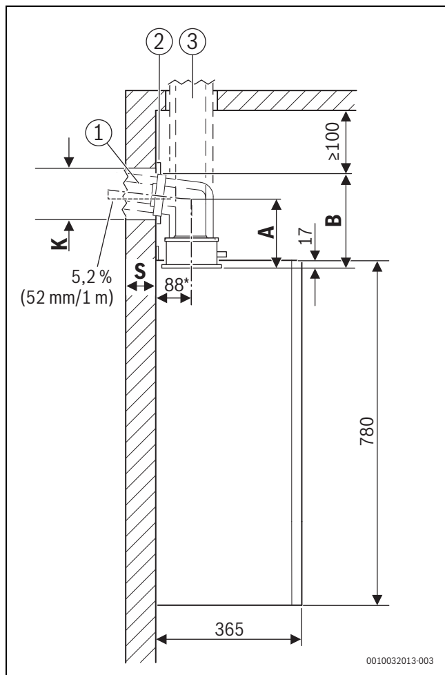
Bild 15 Seitenansicht (Maße in mm)
