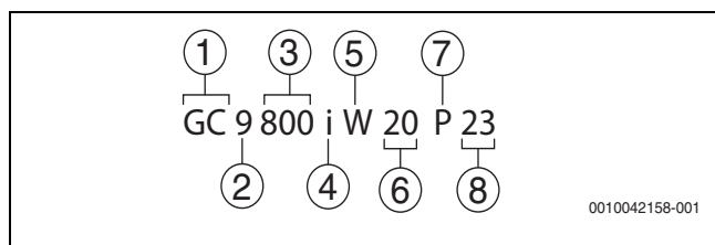
Bild 1 Typenschlüssel
