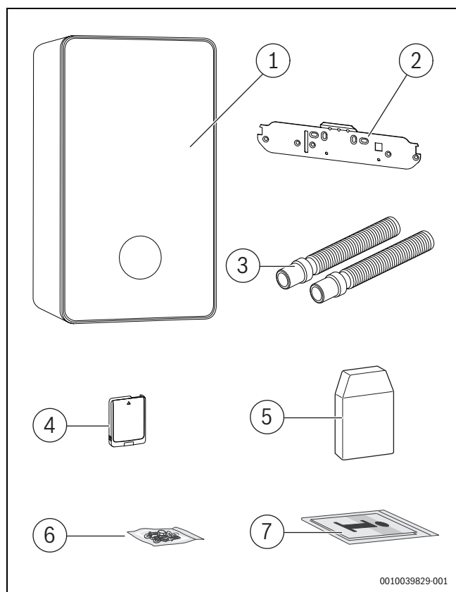
Bild 12 Lieferumfang
