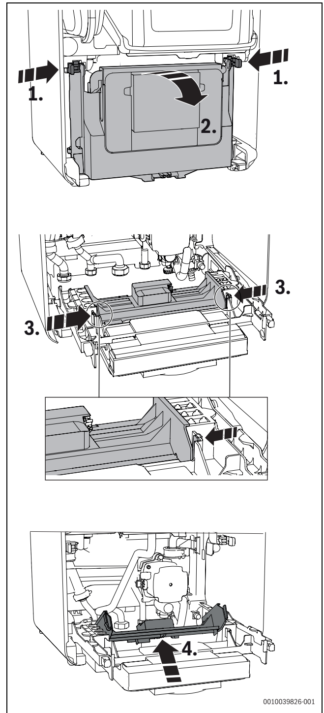
Bild 29 Steuergerät öffnen
