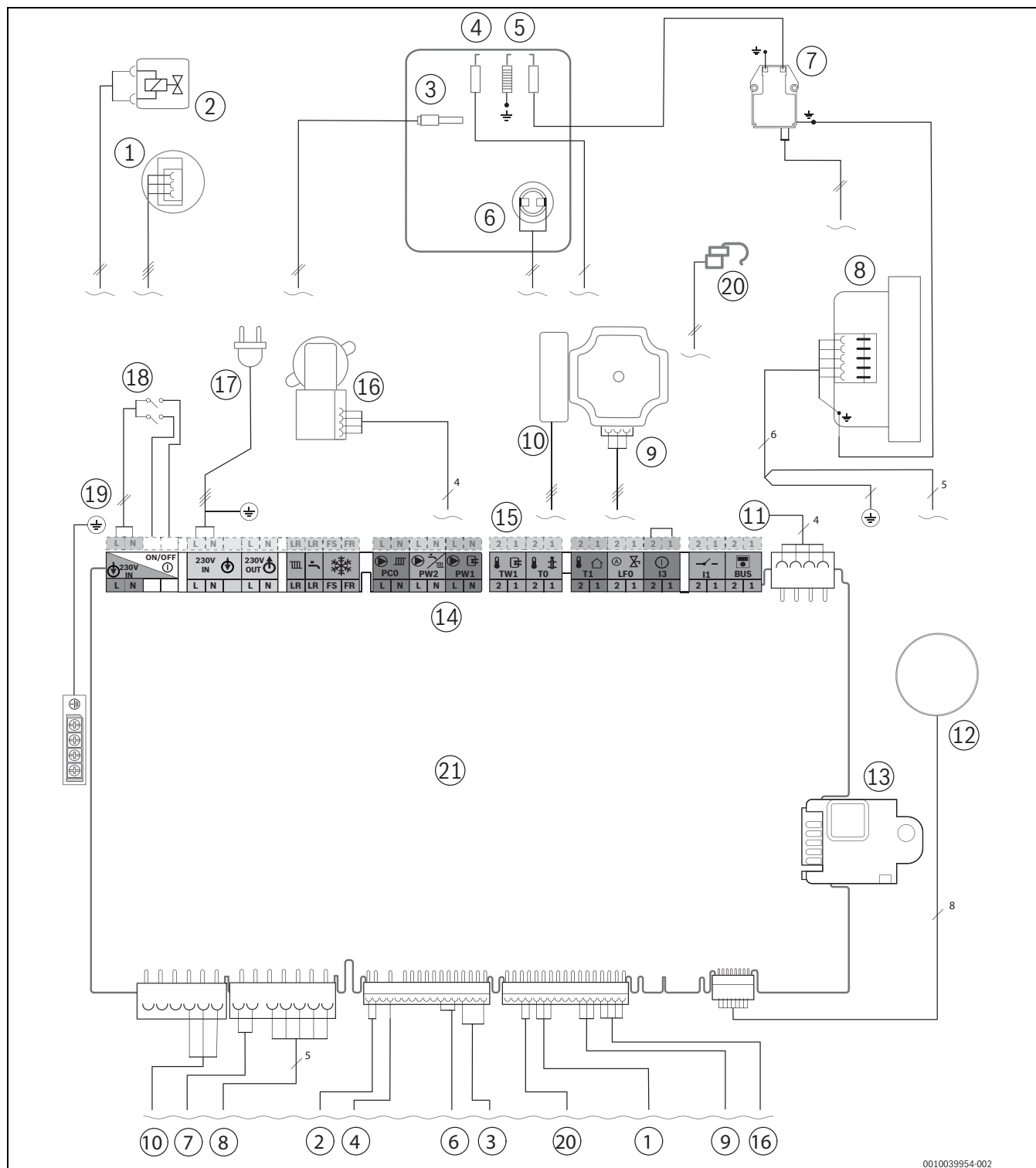
Bild 23 Elektrische Verdrahtung
