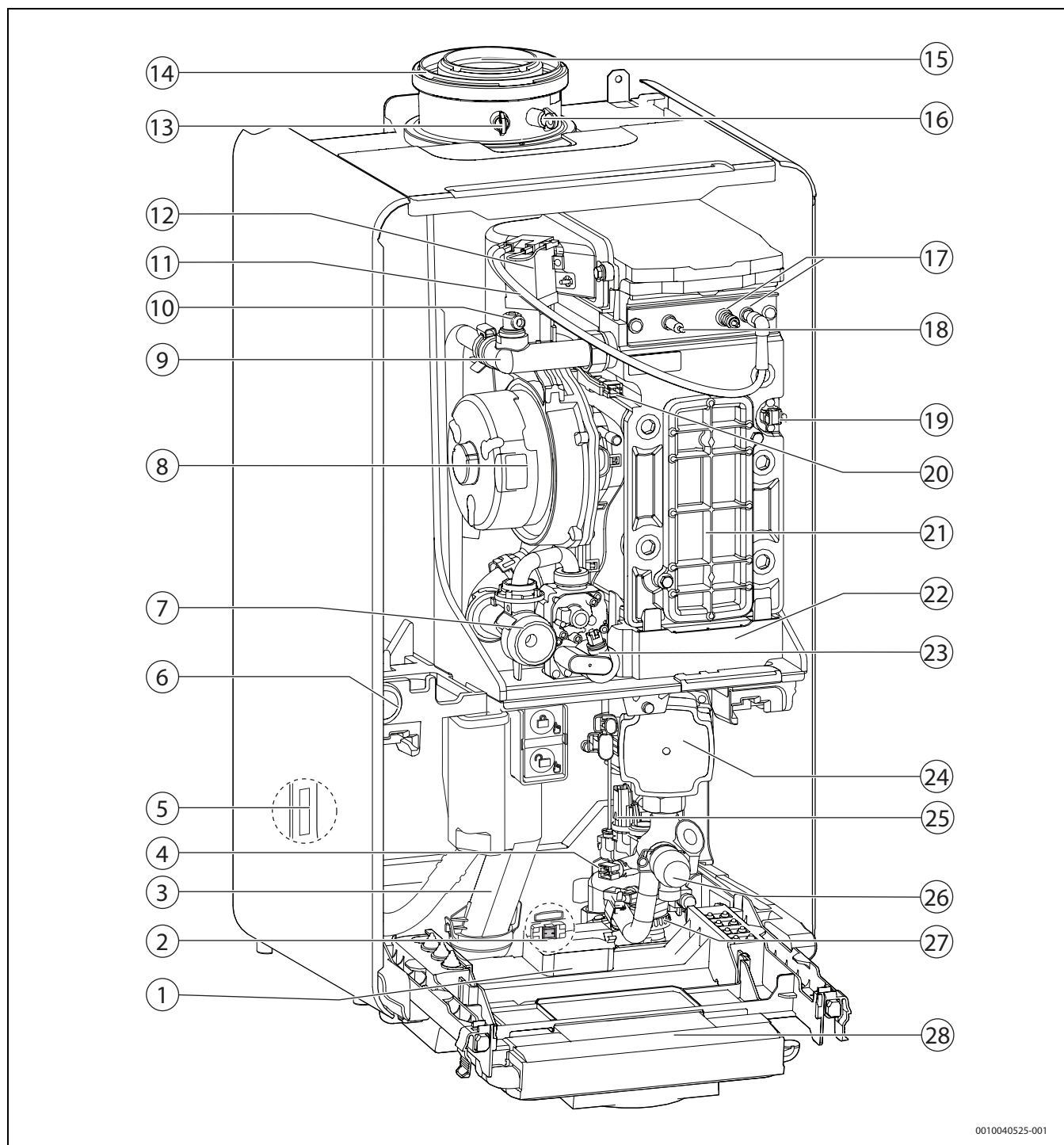
Bild 14 Produktübersicht
