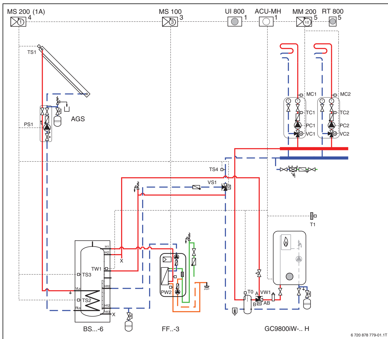
Bild 11 Anlagenschema mit Regelung (unverbindliche Prinzipdarstellung)
