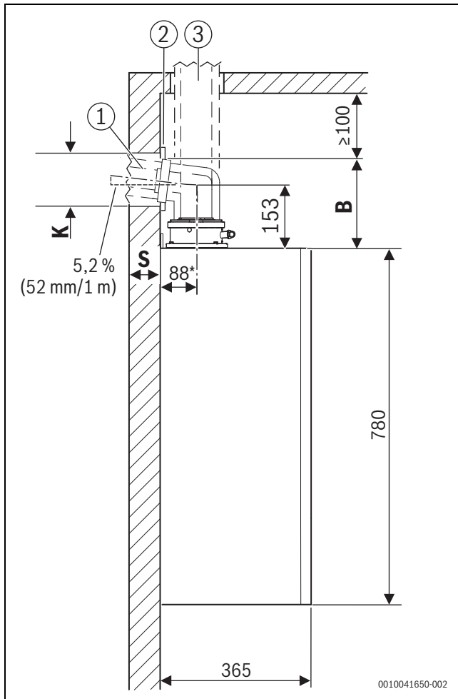
Bild 15 Seitenansicht (mm)
