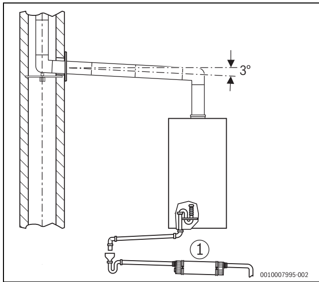
Bild 22 Kondensatschlauch aus dem Gas-Brennwertgerät und eine Kondensatableitung über die Neutralisationseinrichtung
