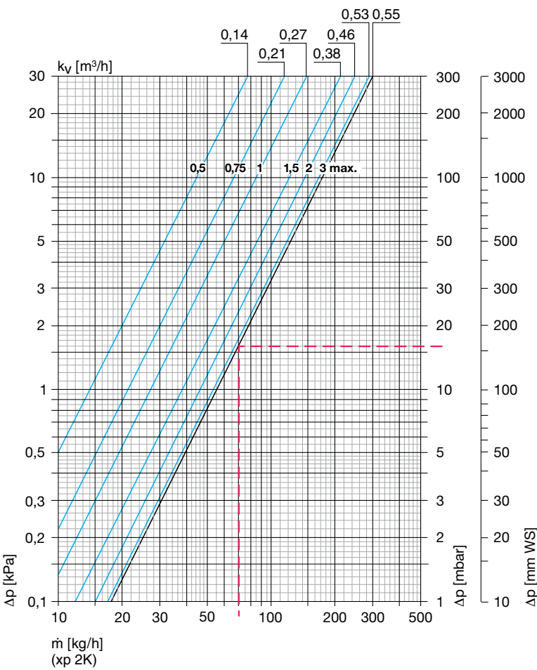
Thermostat-Kopf mit E-Z Ventil Zweirohr
