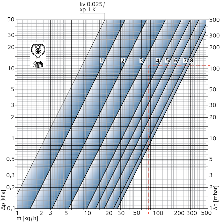
Diagramm, Ventilunterteil mit Thermostat-Kopf
