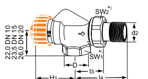
Axial mit verkürzten Baumaßen. Messing. Nicht geeignet für Klemmverschraubungen für Verbundrohr.
